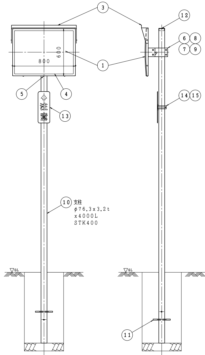
正面図
